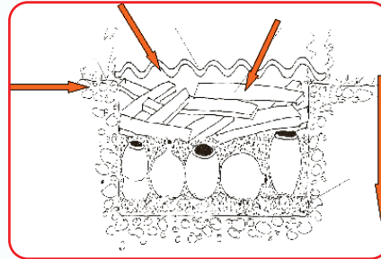
شكل (٦١: ب): الطريقة البدائية الثانية لحرق الأشكال الطينية الجافة في حفرة تحت الأرض.
