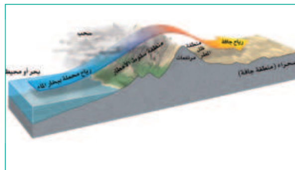
المطر التضاريسي
